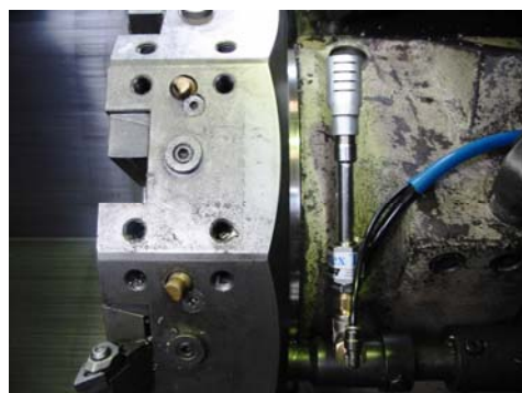
AIR LUBROCOLD installato su tornio CNC con immissione direttamente nel condotto di lubrorefrigerazione della macchina (al posto dell'olio emulsionato)
